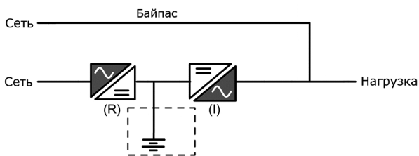
Рисунок 1. Блок-схема
