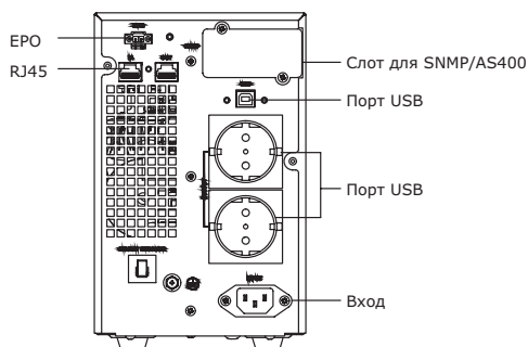
Рисунок 2. Задняя панель модели SMALLB1 (Shucko)
