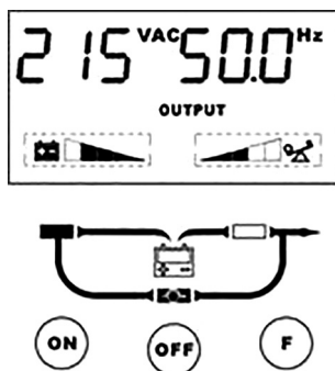
Рисунок 12. Режим байпаса
