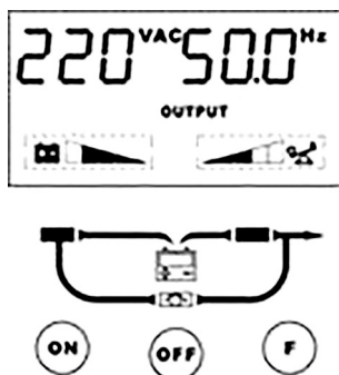
Рисунок 10. Нормальный режим
