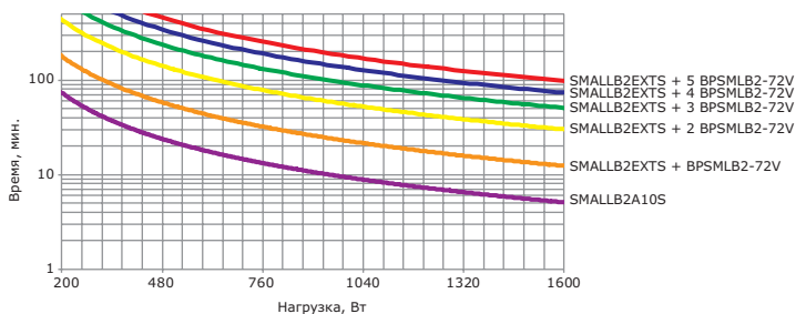
Рисунок 17. График автономной работы ИБП SMALLB2
