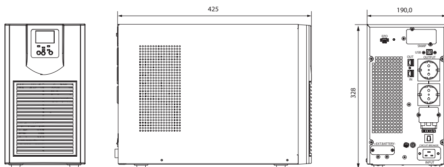
Рисунок 20. Размеры модели SMALLB2 и SMALLB3 (Schuko)
