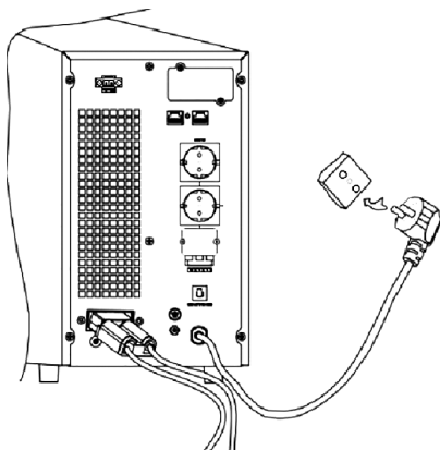
Рисунок 4. Подключение внешних батарейных блоков к ИБП
