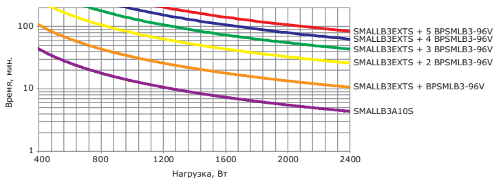
Рисунок 18. График автономной работы ИБП SMALLB3
