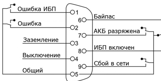
Рисунок 8. Коммуникационный интерфейс AS400
