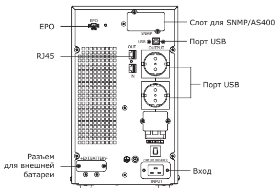
Рисунок 3. Задняя панель моделей SMALLB2 и SMALLB3 (Schuko)
