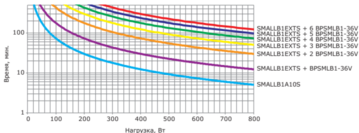
Рисунок 16. График автономной работы ИБП SMALLB1
