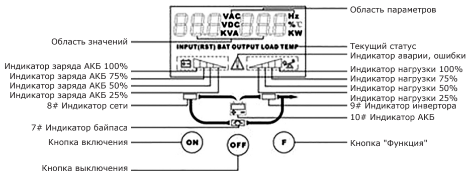
Рисунок 9. Дисплей ИБП
