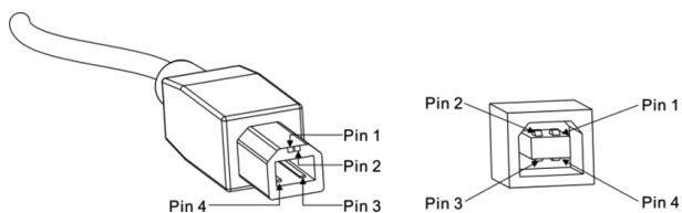
Рисунок 5. Порт USB "папа" (слева), и "мама" (справа)
